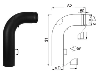
BOCHT, glad, 90°, incl. reinigungsopening en klep
