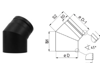
Bocht, vast, 45°, zonder reinigungsopening
