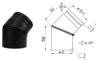
Bocht, draaibaar, 2 delen, 0- 45°, zonder reinigungsopening Bocht, haaks, 2 delen, 90°, incl. reinigungsopening en klep
