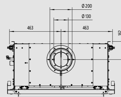
Zijaanzicht
