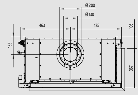
Zijaanzicht
