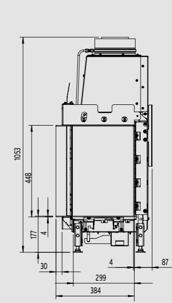
Zijaanzicht
