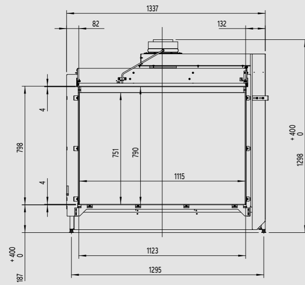
Bovenzijde
