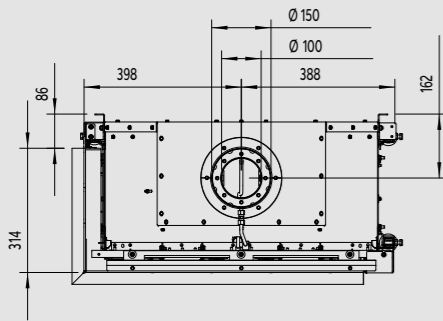
Zijaanzicht
