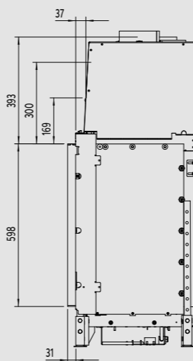
Zijaanzicht
