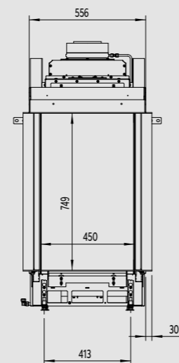
Zijaanzicht
