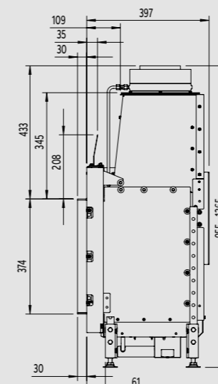
Zijaanzicht
