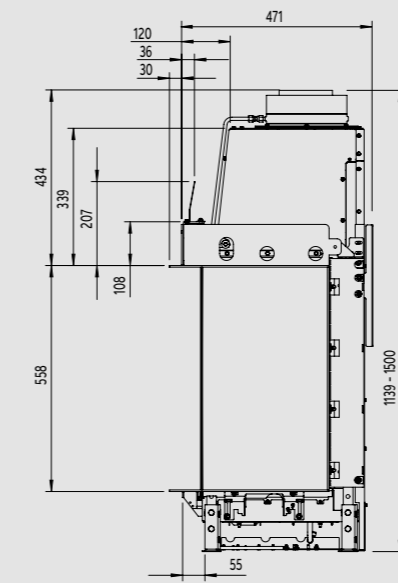
Zijaanzicht
