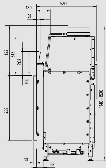
Zijaanzicht
