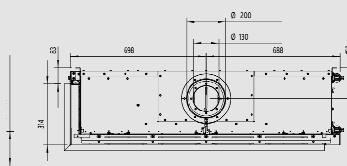
Zijaanzicht
