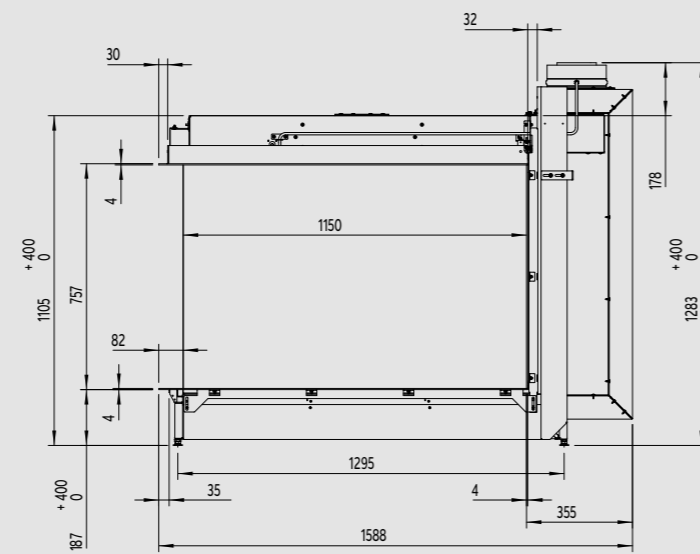
Bovenzijde
