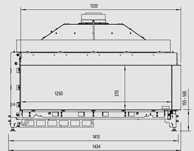
Bovenzijde
