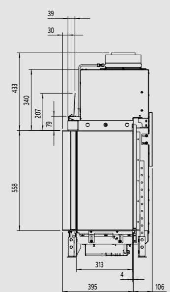
Zijaanzicht
