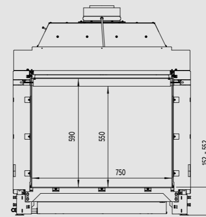
Bovenzijde
