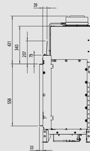
Zijaanzicht
