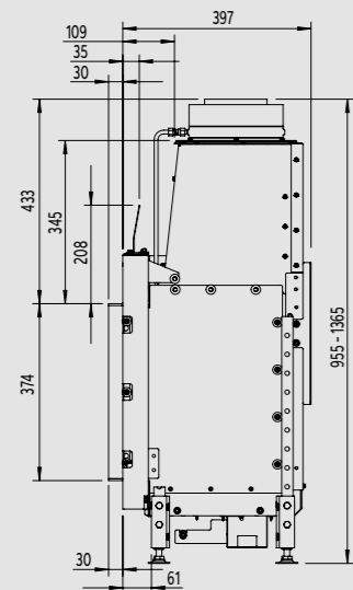
Zijaanzicht
