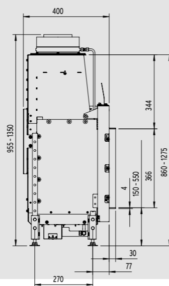
Zijaanzicht
