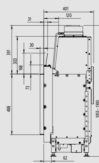
Zijaanzicht
