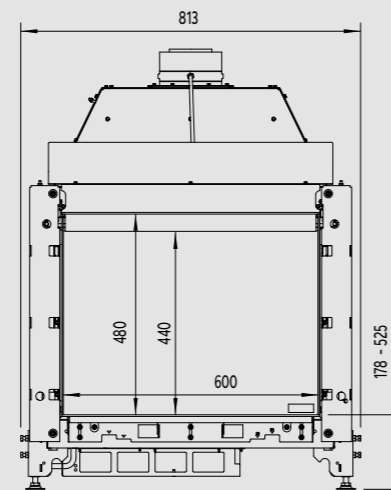
Bovenzijde
