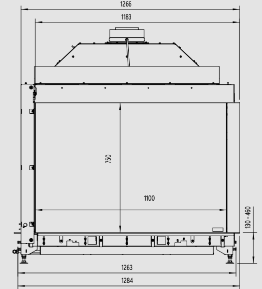
Bovenzijde
